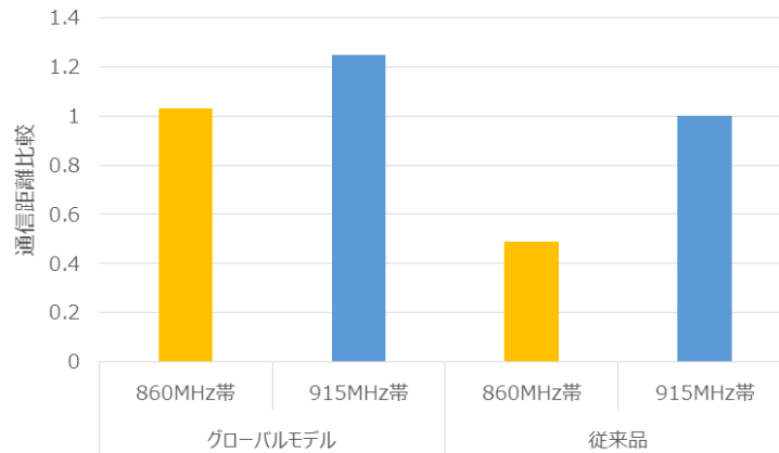
通信性能比較グラフ
